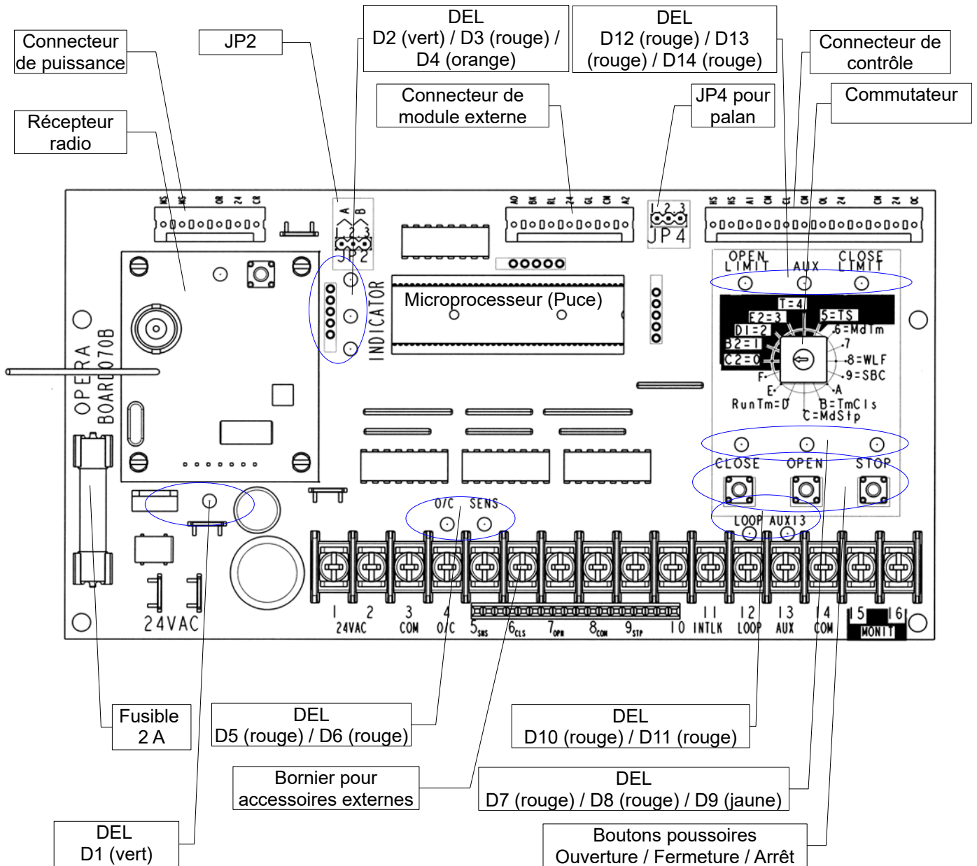
Figure 34 - Circuit de contrôle électronique – BOARD 070M
