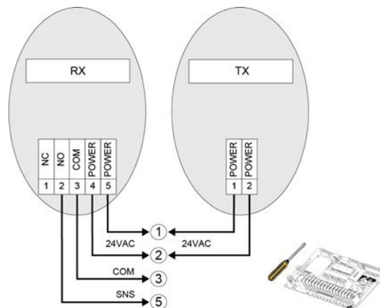
Figure 22 - PHOTO 015 / 016 / 045 / 050 / 051 / 059
