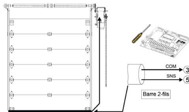
Figure 29 - Barre palpeuse électrique
