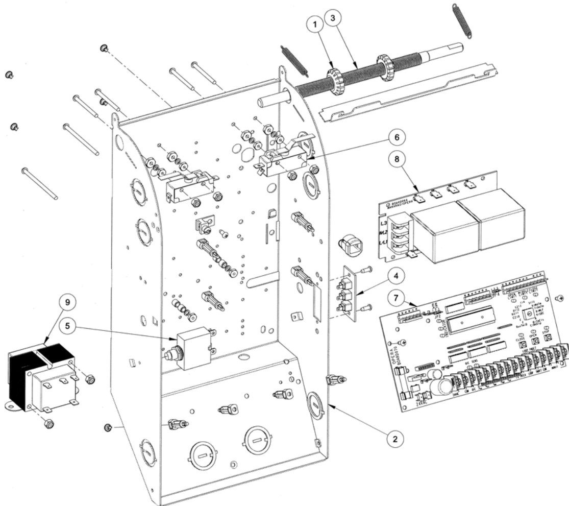
Figure 42 - Enceinte de contrôle OTH / OTBH / MGT avec BOARD 070M
