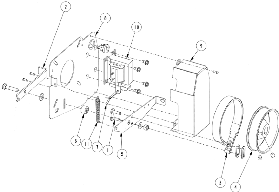
Figure 41 - Vue explosée BRAKE 011
