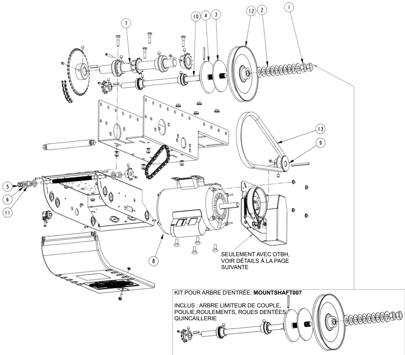
Figure 40 - Vue explosée OTH / OTBH
