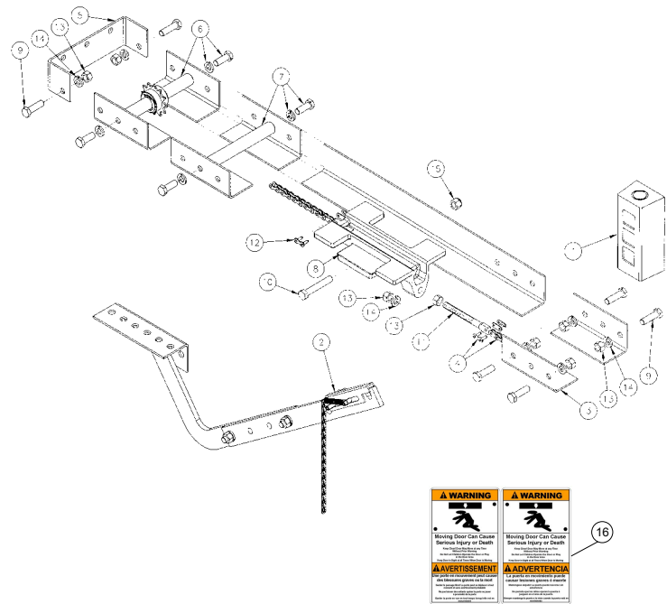
Figure 3 - Quincaillerie standard pour opérateur aérien
