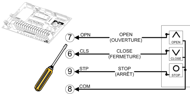
Figura 17 - STATION 020 / 084 (estación) 3-PBS Abrir / Cerrar / Detener
