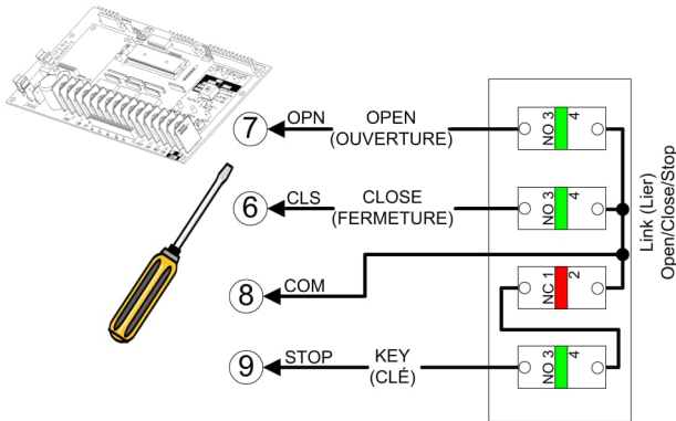
Figura 19 - STATION 079 (estación) 3-PBS Abrir / Cerrar / Detener con Llave
