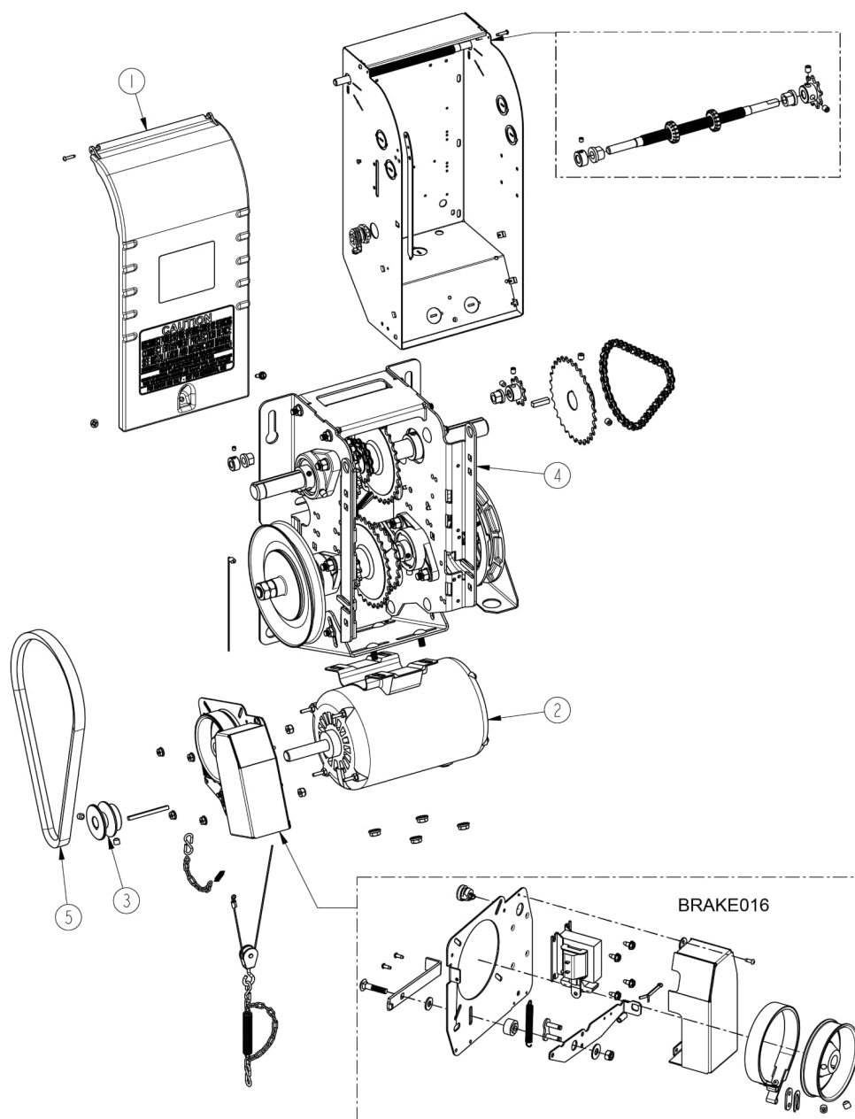
Figura 50 - Despiece mecánico Rapido RSH/RVH
