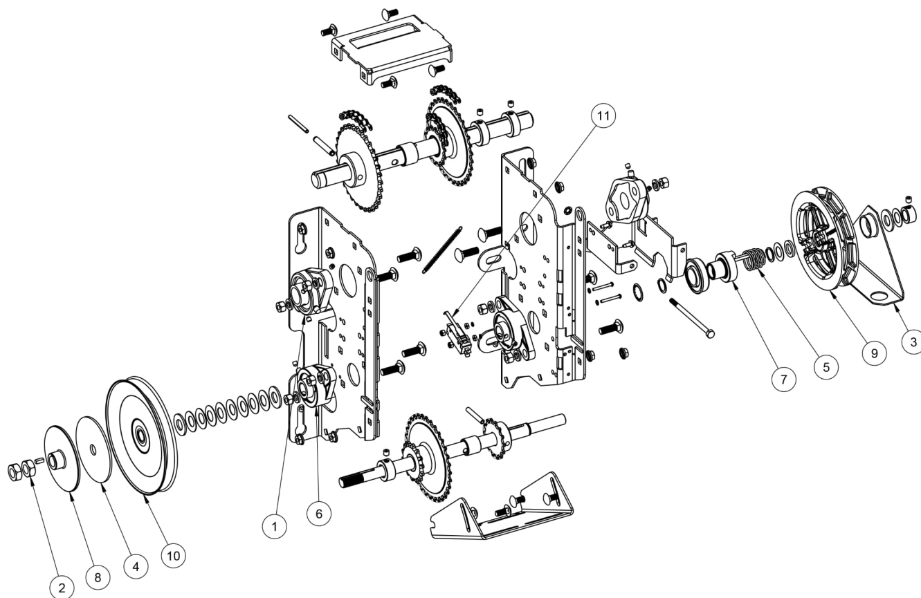
Figura 51 - Despiece mecánico del subconjunto estructura-reducción de Rapido RSH/RVH
