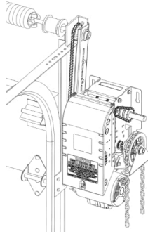
Figura 5 - Montaje de pared lado derecho (polea de cadena a la derecha)
