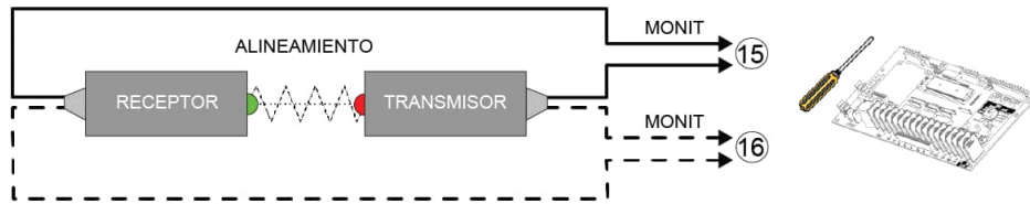
Figura 26 - SENSEEDGE042 instalación
