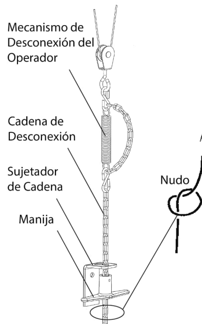
Figura 11 - Cadena de desconexión
