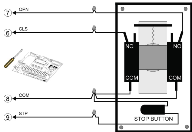
Figura 41 - KEYSWITCH 019 (Interruptor de llave)
