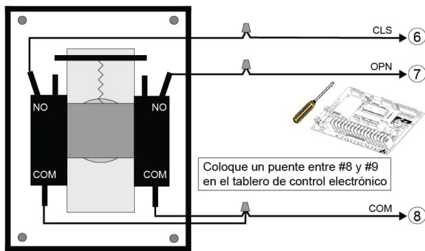
Figura 40 - KEYSWITCH 010 / 015 (Interruptor de llave)
