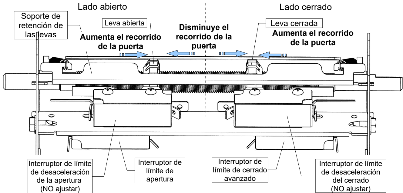
Figura 13 - Ajuste de los interruptores y de las levas de límite
