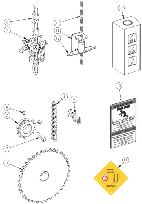
Figura 2 - Hardware para eje de transmisión estándar
