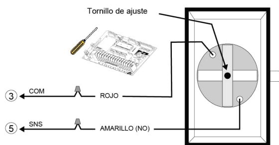
Figura 36 - AIRSWITCH 001 / 007 (Interruptor de aire)
