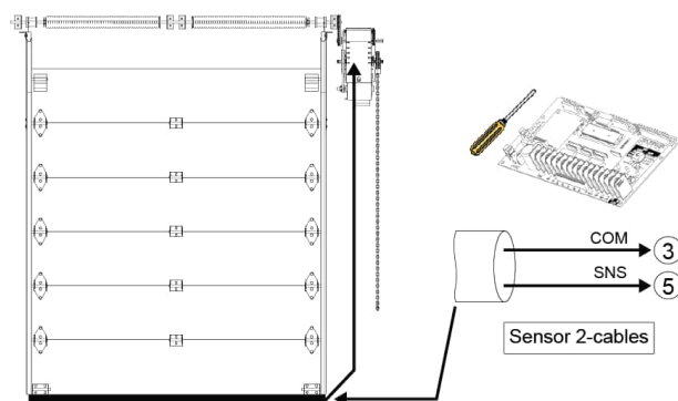
Figura 38 - Borde de detección eléctrico
