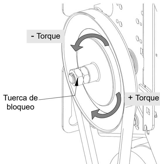
Figura 45 - Ajuste del embrague
