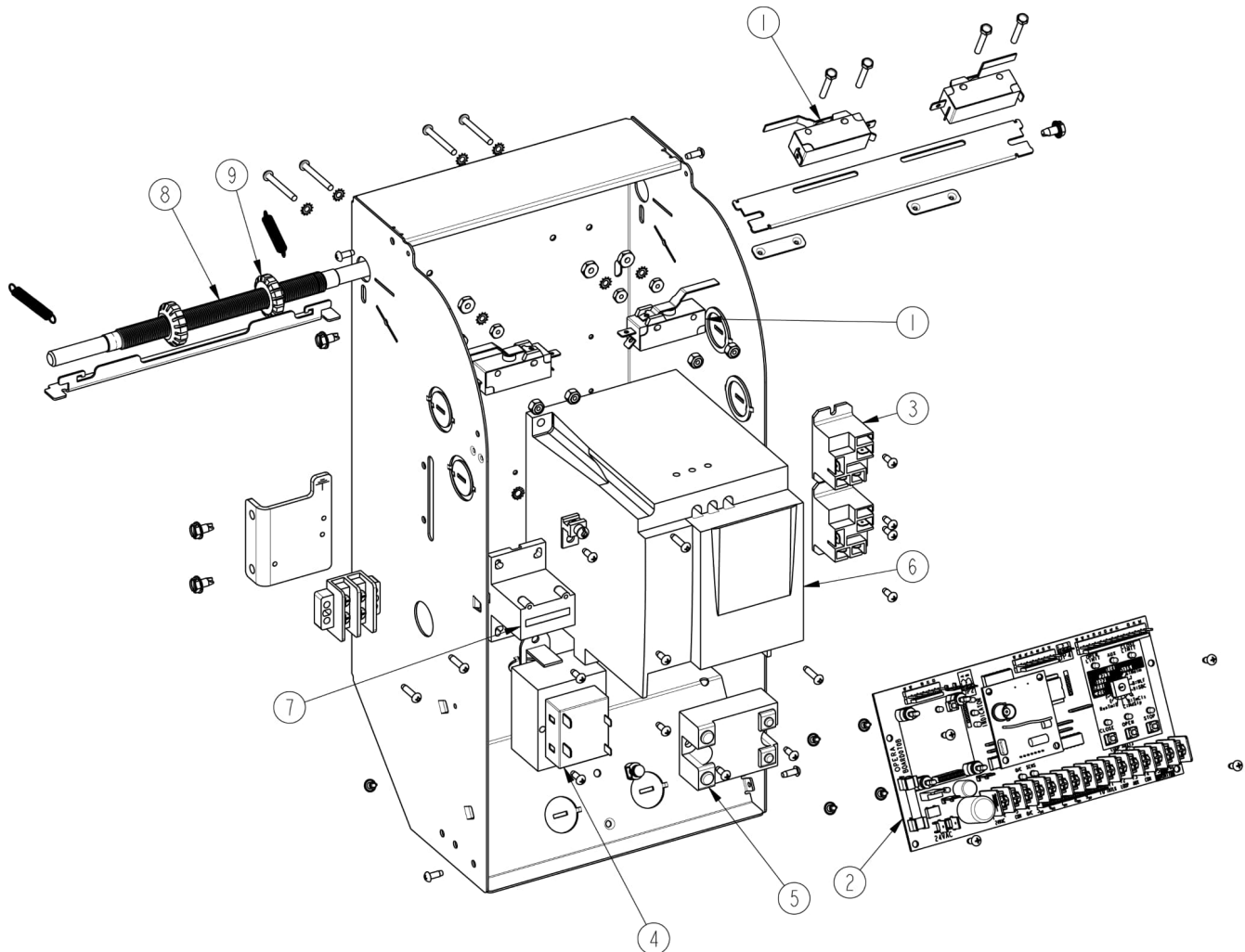
Figura 53 - Caja de control Rapido RGH/RMSJ/RSH/RTBH/RVH 115VAC con BOARD 070M
