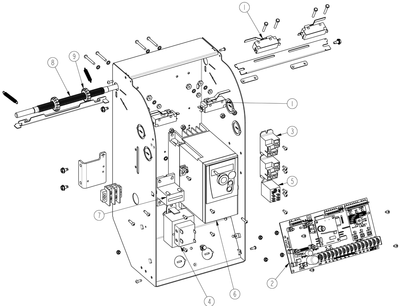
Figura 54 - Caja de control de Rapido RGH/RMSJ/RSH/RTBH/RVH 208/230VAC con BOARD 070M
