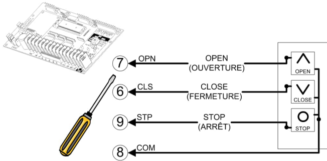
Figura 17 - STATION 020 / 084 (estación) 3-PBS Abrir / Cerrar / Detener
