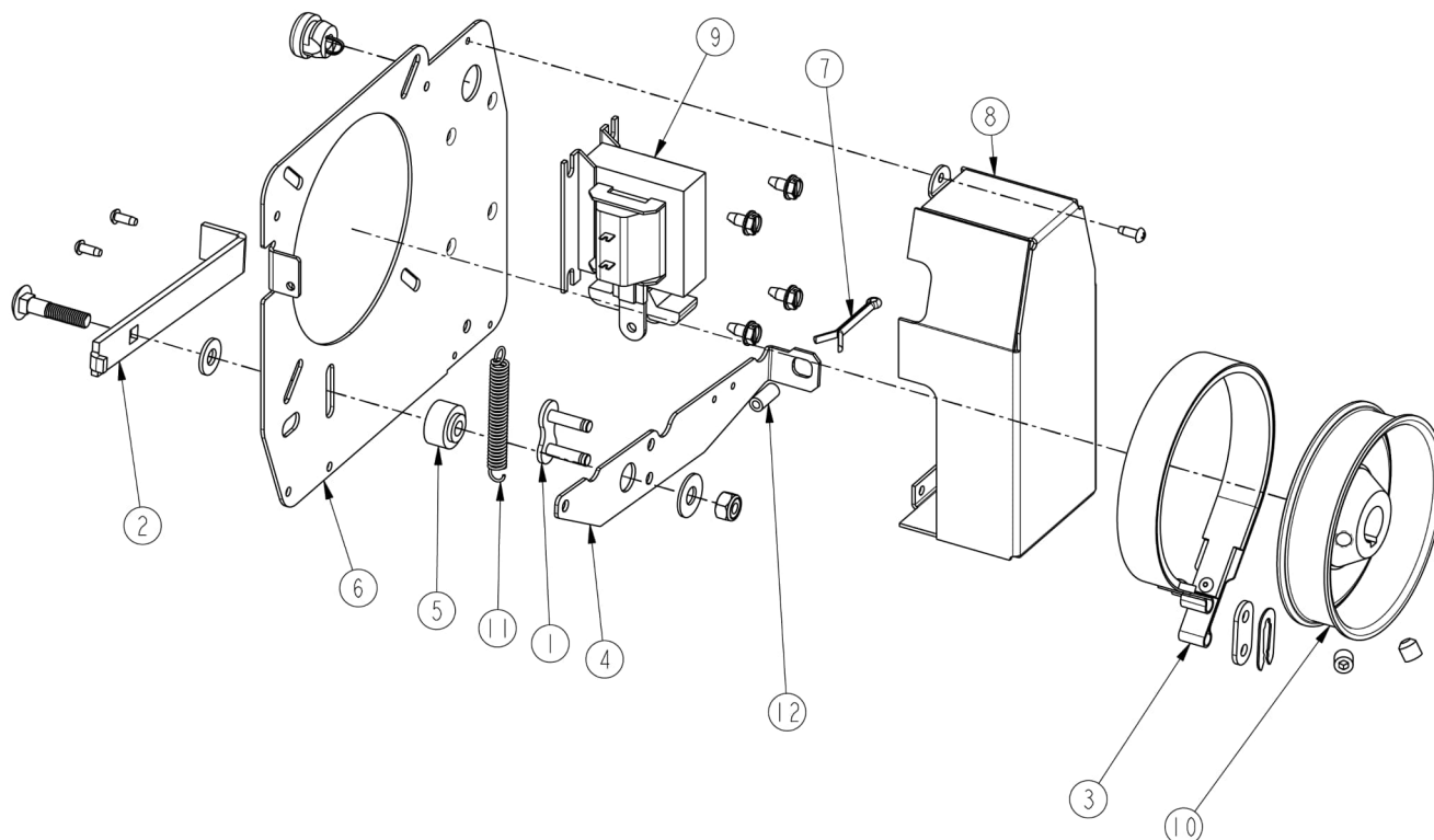
Figura 52 - Despiece mecánico de BRAKE 016
