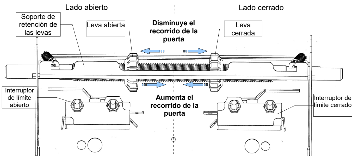
Figura 13 - Ajuste de límite de carrera
