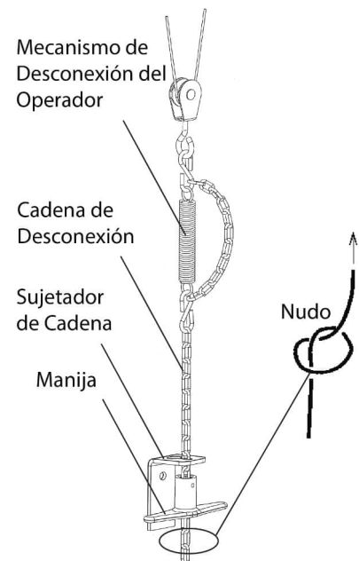
Figura 11 - Cadena de desconexión
