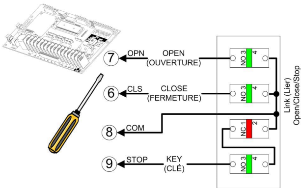
Figura 17 - STATION 079 (estación) 3-PBS Abrir / Cerrar / Detener con Llave
