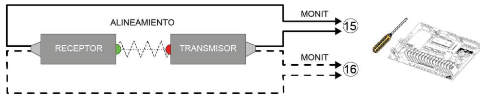
Figura 21 - PHOTO 061 / 061A / 070 instalación
