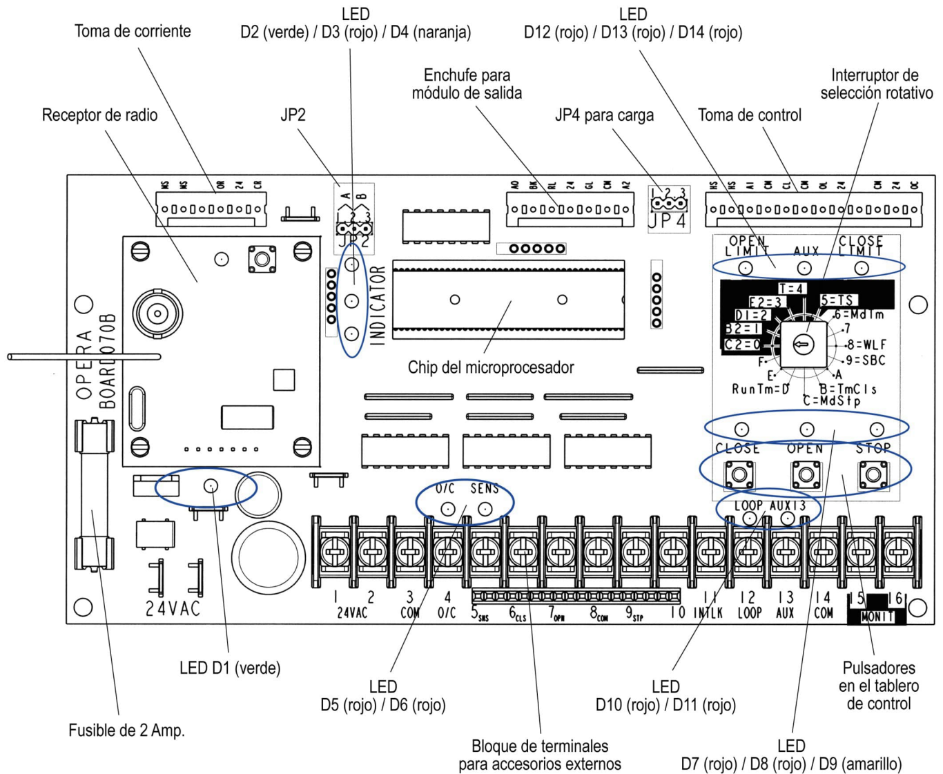
Figura 41 - Tablero de control electrónico – BOARD 070M
