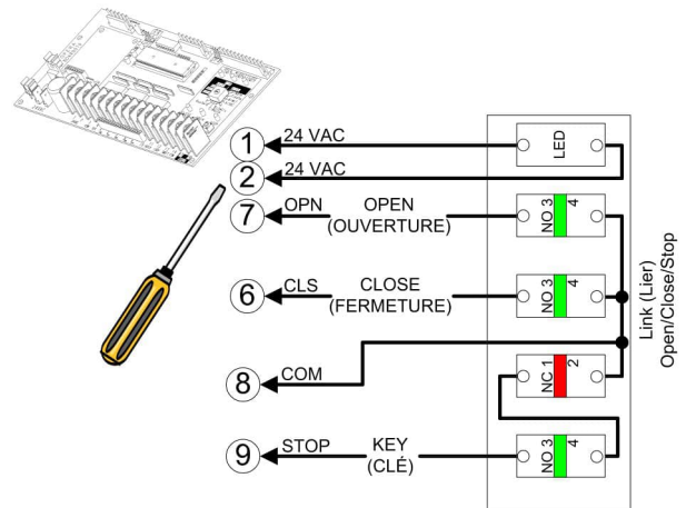
Figura 18 - STATION 080 (estación) 3-PBS Abrir / Cerrar / Detener con Llave y Luz
