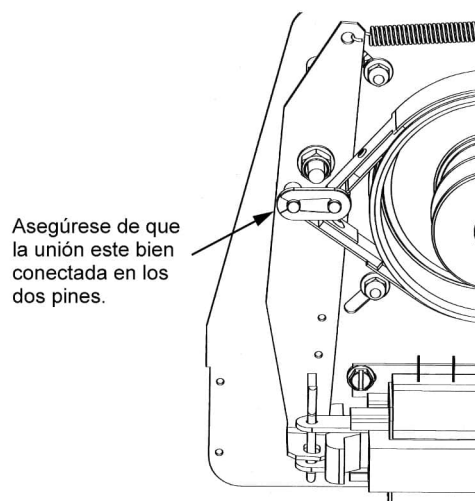
Figura 44 - Procedimiento de reemplazo de la banda de freno
