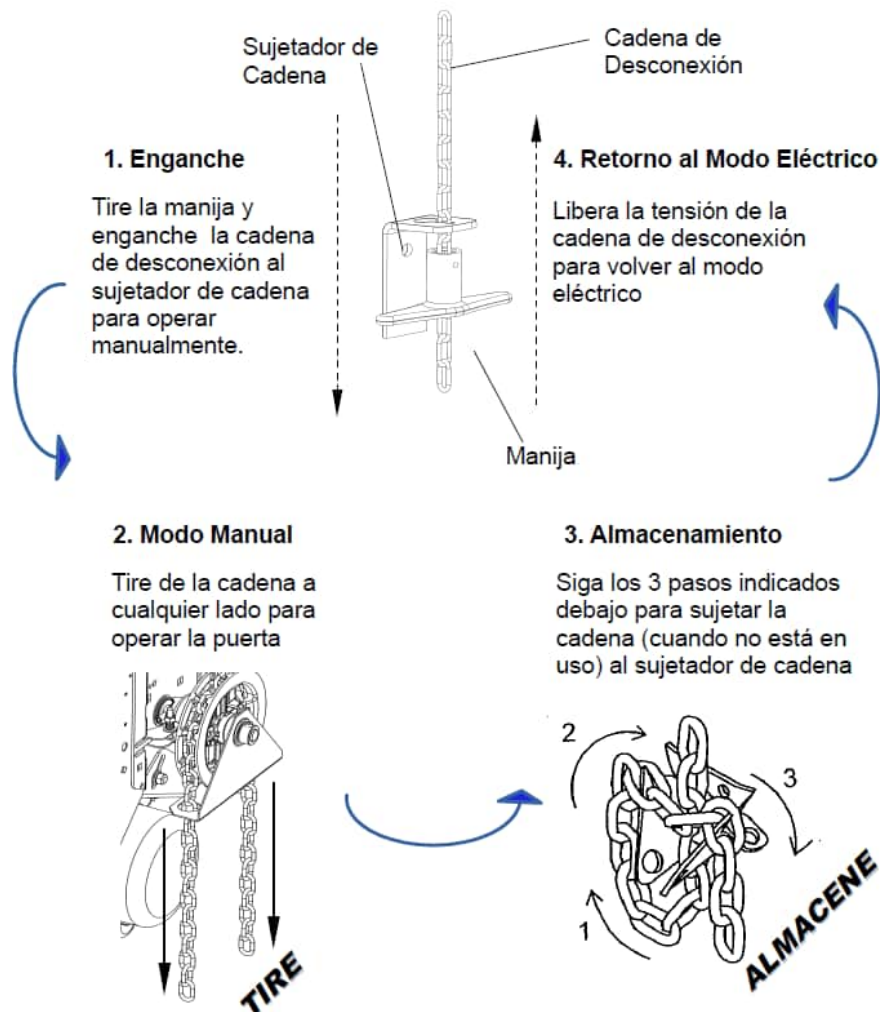
Figura 12 - Enganche y operación de la polea
