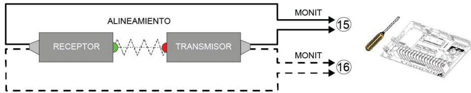
Figura 24 - SENSEEDGE042 instalación
