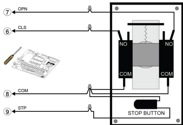
Figura 39 - KEYSWITCH 019 (Interruptor de llave)
