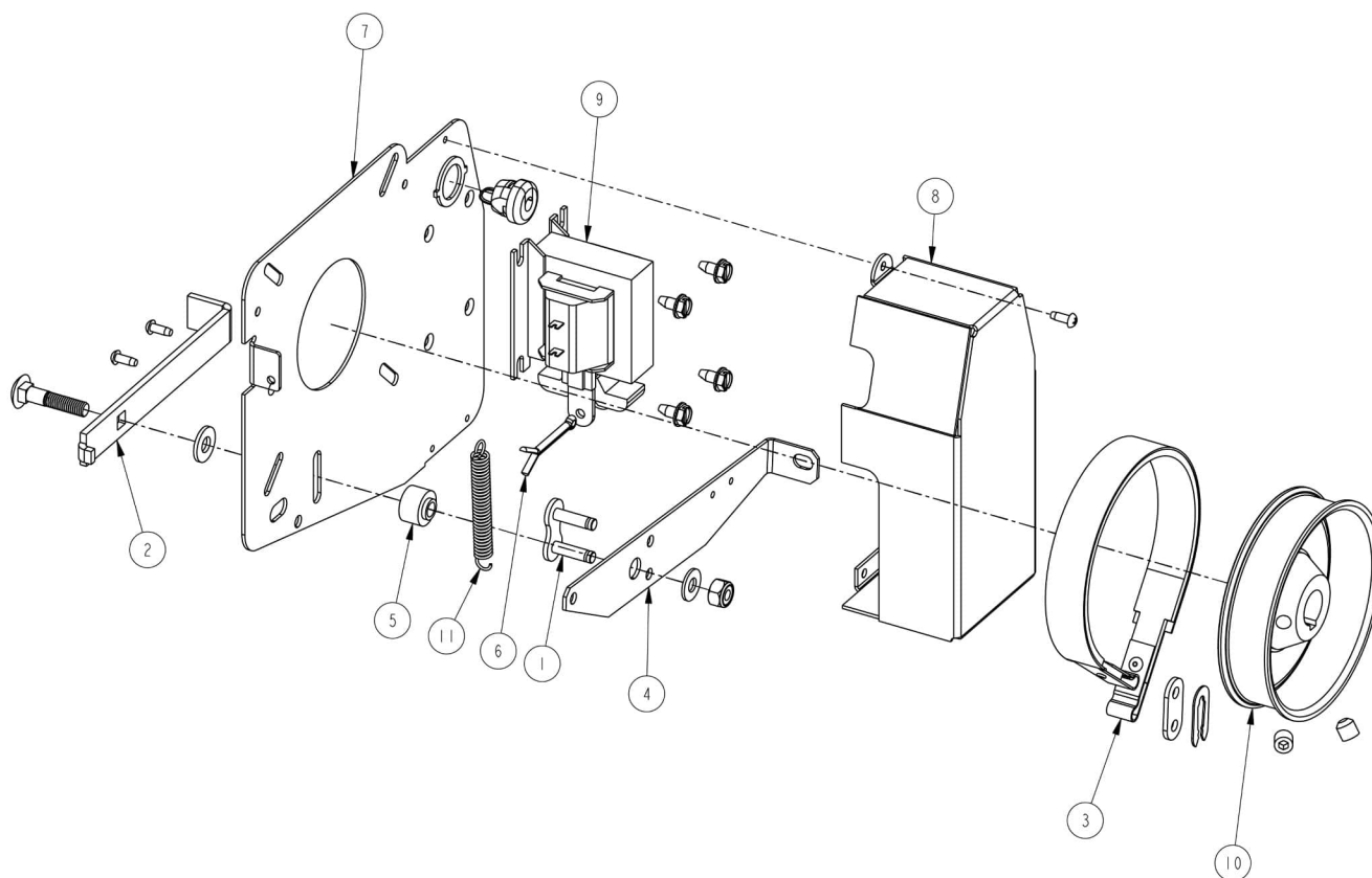
Figura 51 - Despiece mecánico de BRAKE 013
