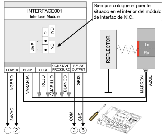
Figura 28 - PHOTO 008D1 / D2 (celdas fotoeléctricas)
