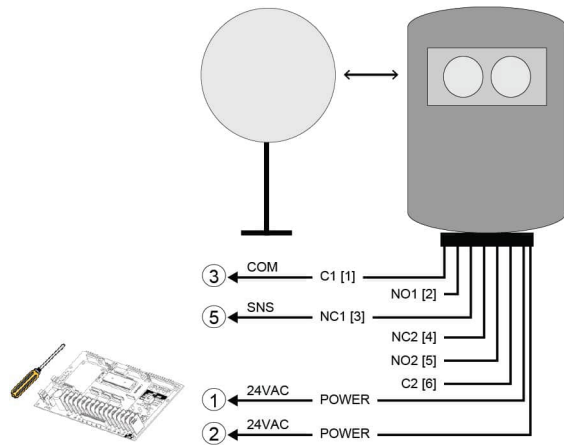
Figura 31 - PHOTO 018 (celdas fotoeléctricas)
