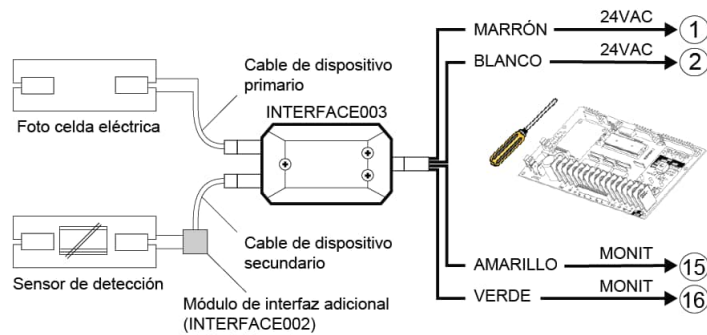
Figura 26 - INTERFACE 003 instalación
