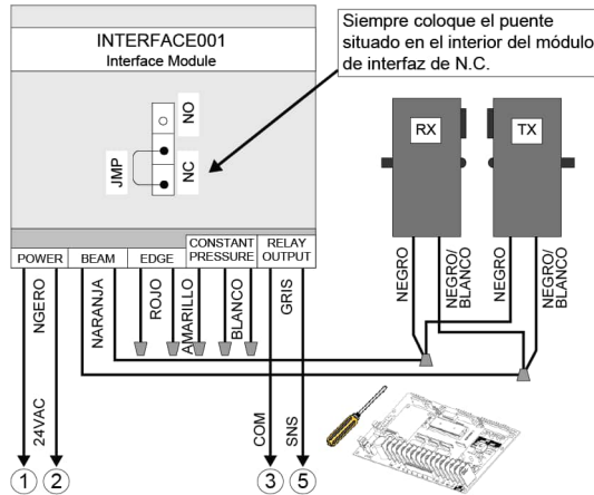
Figura 27 - PHOTO 008C3 / C4 / E1 (celdas fotoeléctricas)
