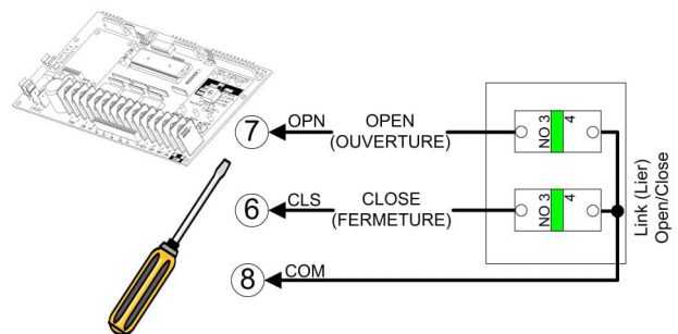
Figura 20 - STATION 010 / 082 (estación) 2-PBS Abrir / Cerrar
