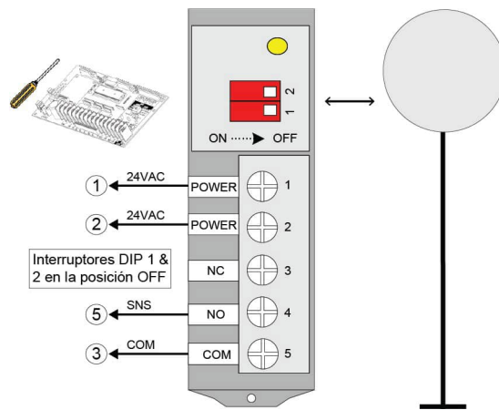
Figura 30 - PHOTO 060 (celdas fotoeléctricas)
