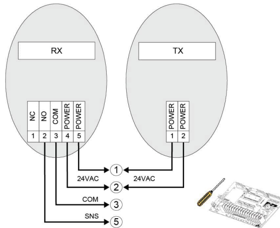
Figura 29 - PHOTO 015 / 016 / 045 / 050 / 051 / 059 (celdas fotoeléctricas)
