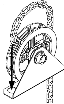
Figura 10 - Instalación de la cadena en la polea
