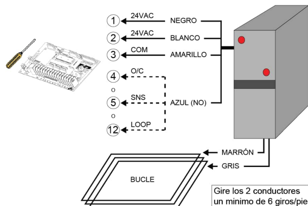
Figura 40 - Detector de bucle de vehículo
