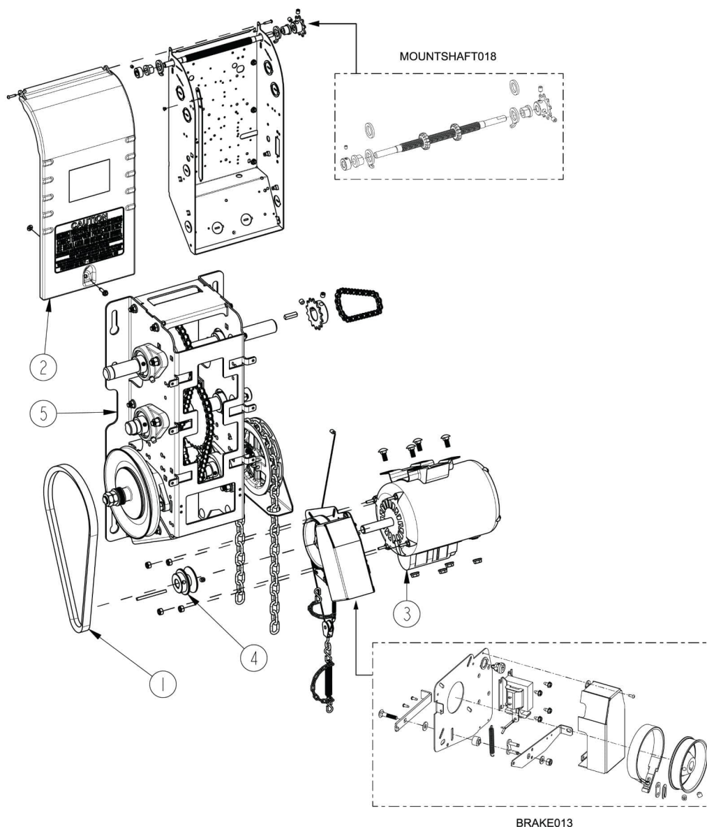
Figura 49 - Despiece mecánico de MSJ
