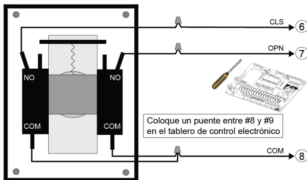
Figura 38 - KEYSWITCH 010 / 015 (Interruptor de llave)
