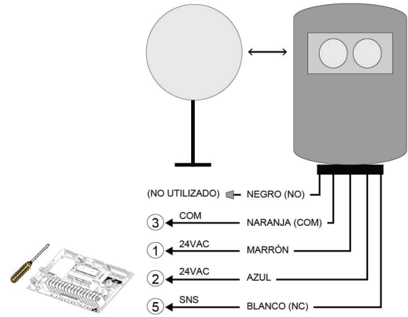
Figura 32 - PHOTO 038 (celdas fotoeléctricas)
