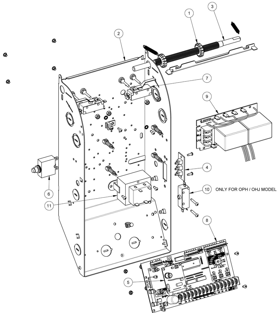
Figura 52 - Caja de control Opera con tablero de control electrónico BOARD070M/E
