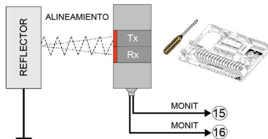
Figura 22 - Instalación de PHOTO 065
