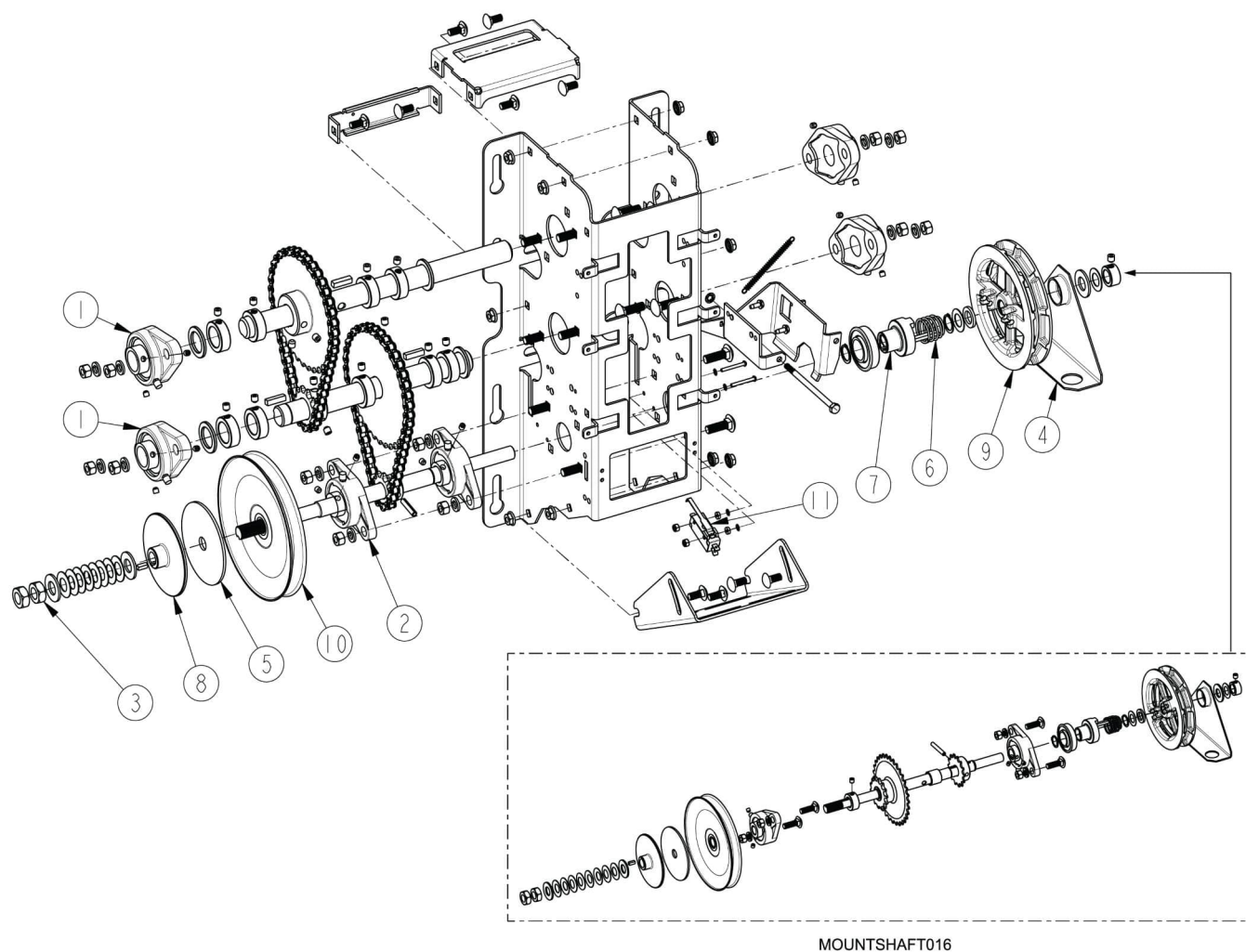
Figura 50 - Despiece mecánico del subconjunto estructura-reducción de MSJ
