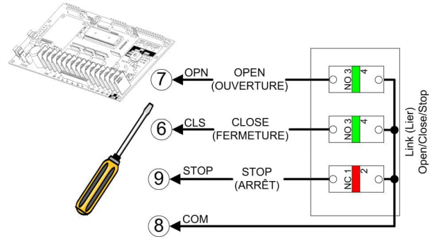
Figura 16 - STATION 041 / 049 / 056 / 076 / 078 (estación) 3-PBS Abrir / Cerrar / Detener
