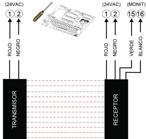
Figura 25 - LIGHTCURTAIN 001 / 002 instalación
