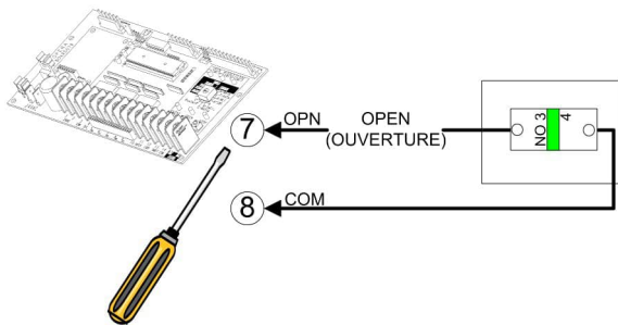
Figura 19 - STATION 001 / 081 (estación) 1-PBS Abrir
