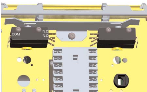
Ancienne configuration du système de fins de courses >>>
