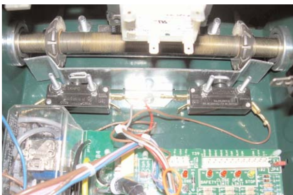
Ancienne configuration du système de fins de courses >>>
